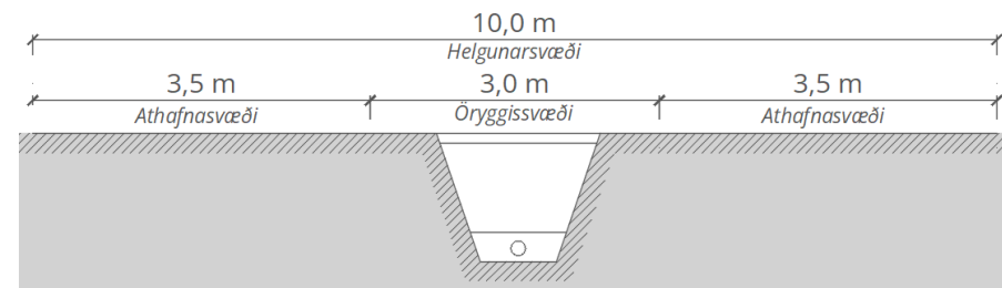
Mynd 3.3: Helgunarsvæði jarðstrengja skiptist í öryggissvæði og athafnasvæði sbr. leiðbeiningar Landsnets um öryggisreglur vegna vinnu í námunda við háspenna jarðstrengi.
