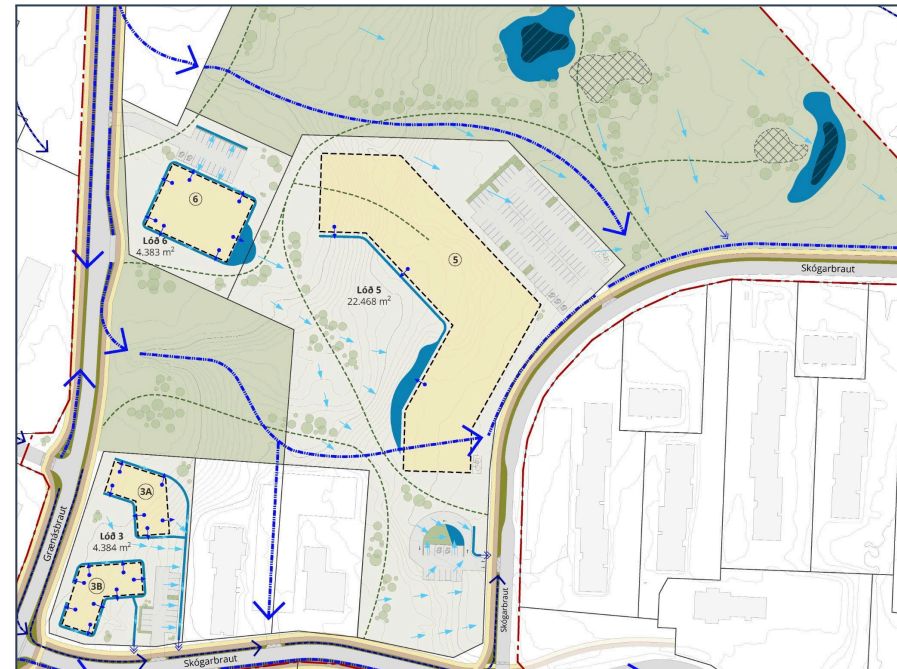
Mynd 3.10: Meginlínur um fyrirkomulag blágrænna ofanvatnslausna á lóð 5 og 6.
