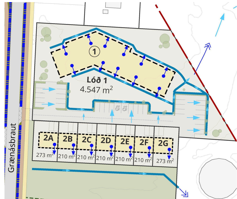
Mynd 3.8: Meginlínur um fyrirkomulag blágrænna ofanvatnslausna á lóð 1 og 2A-2G.
